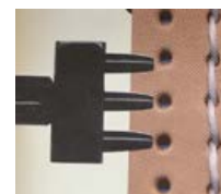
3201-03 Perforateur 3 trous ronds couture à la main / 3 round hole punch for hand stitching 1,5 mm X 3 mm
